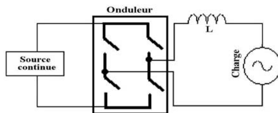
Fig. 2: Montage de base d'un onduleur photovoltaïque
