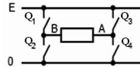
Fig. 6: Pont de puissance a transistor
