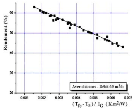
Capteur avec chicanes – 65 m³/h
