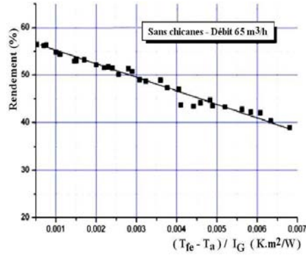
Capteur sans chicanes – 65 m³/h
