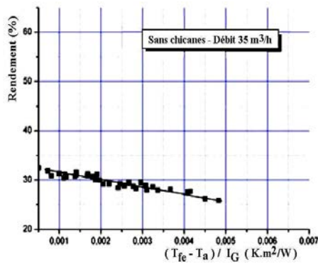
Capteur sans chicanes – 35 m³/h
