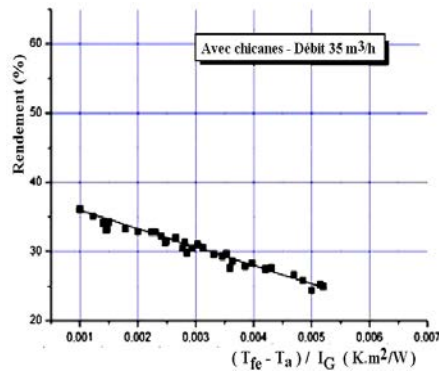
Capteur avec chicanes – 35 m³/h
