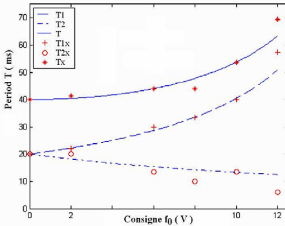
Fig. 9: Durées d'impulsions en fonction de f_0
