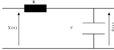
Fig. 3: Filtre passe bas de 1 er ordre
