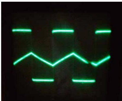
Fig. 8: Images de l'oscilloscope montrant U(t) et Z(t)
