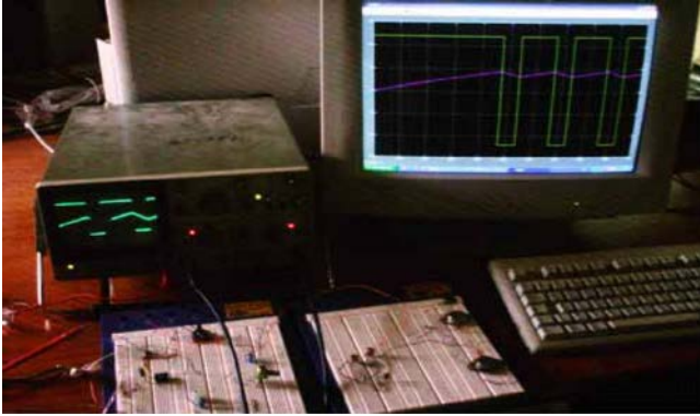
Fig. 7: Système expérimental
