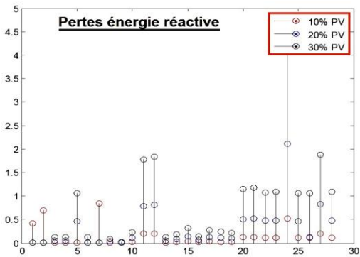
Fig. 4: Pertes énergie réactive
