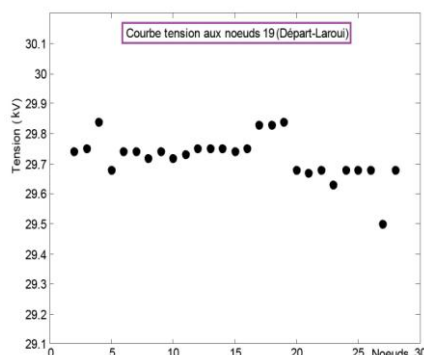
Fig. 12: Tension au nœud 19 (Dép. Laroui)
