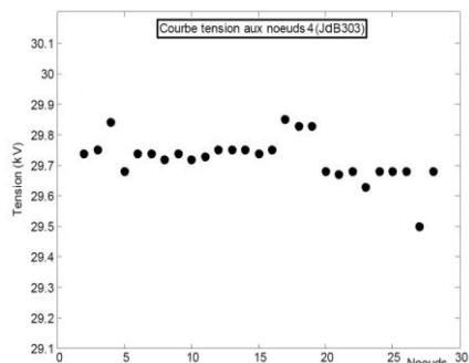
Fig. 8: Tension au nœud 4 (JdB303)
