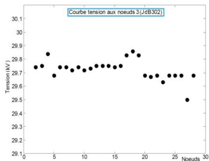
Fig. 7: Tension au nœud 3 (JdB302)
