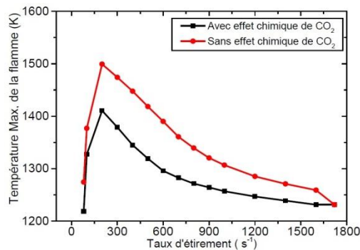
Fig. 9: Effet chimique du CO 2 sur la température pour différents taux d'étirement
