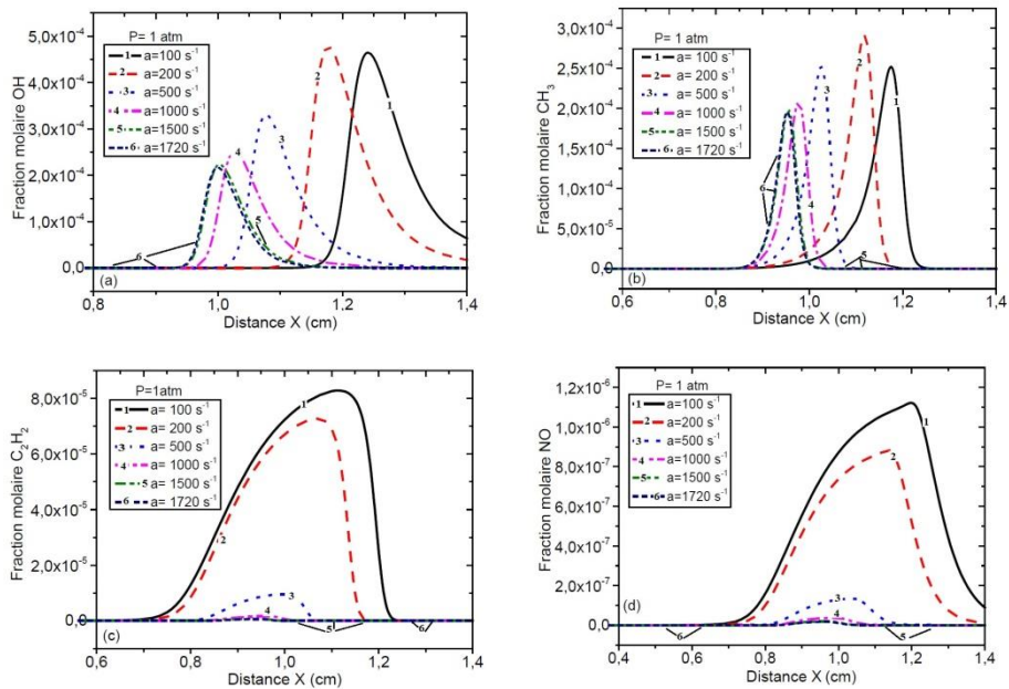
Fig. 8: Fraction molaire des espèces pour différents taux d'étirement
