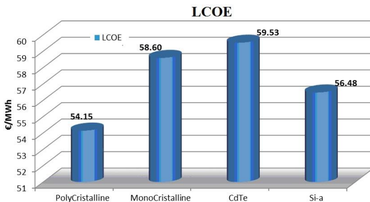
Fig. 6: Coût unitaire de l'énergie produite (LCOE)
