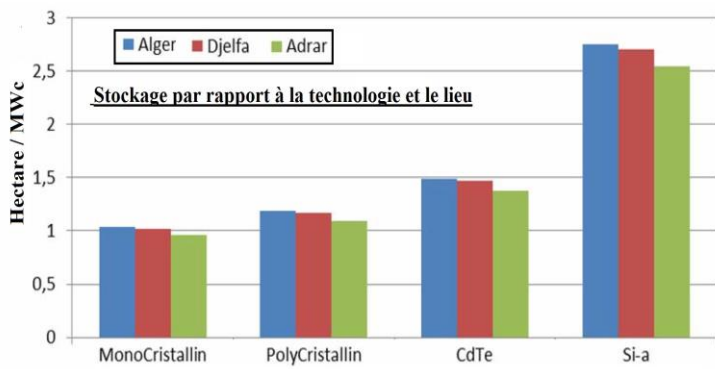
Fig. 3: Estimation de la surface occupée par les centrales PV
