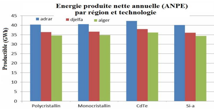
Fig. 4: Energie produite nette annuelle
