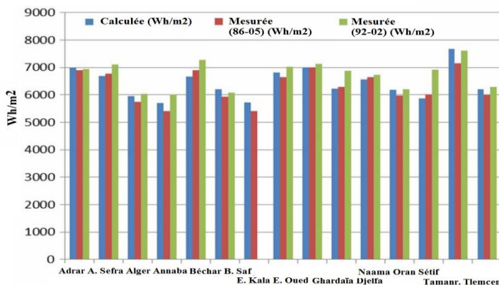
Fig. 2: Potentiel solaire en Algérie
