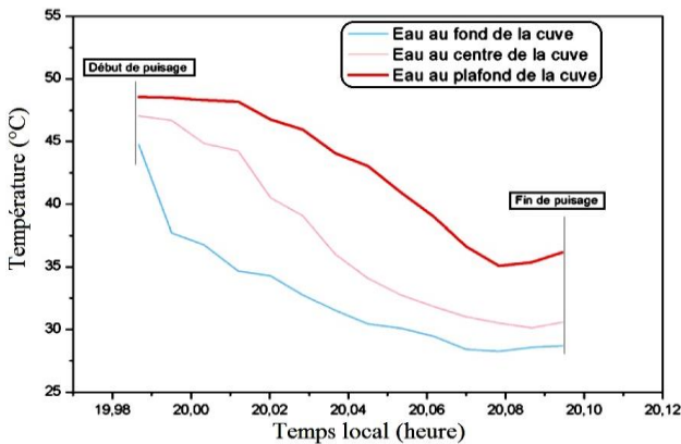
Fig. 13: Stratification de l'eau chaude à l'intérieur de la cuve pendant le puisage d'eau avec un débit de l'ordre de (05) l/mn lors de la journée du 25 Janvier 2018
