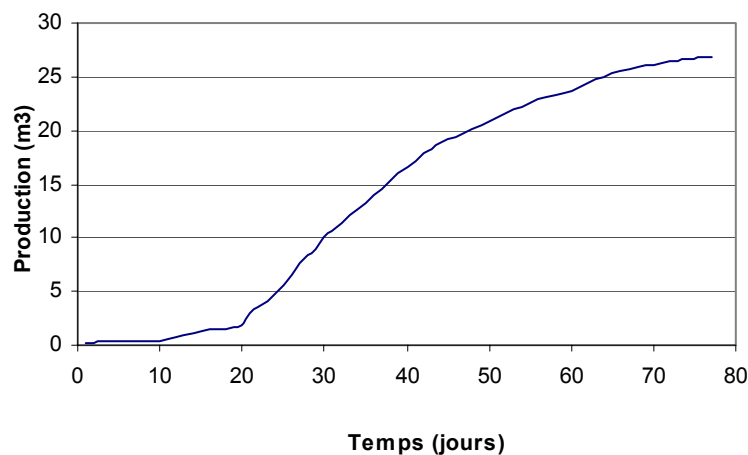
Fig. 2: Cinétique de la production cumulée du biogaz
