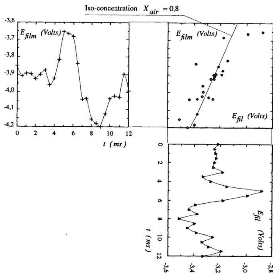
Fig. 5: Visualisation des signaux délivrés par le fil et le film.
