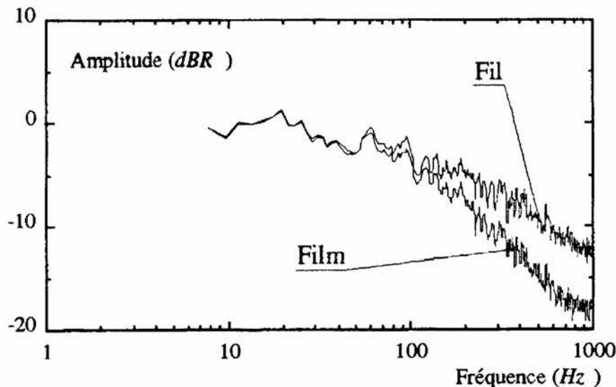
Fig. 6: Spectres de tension du fil et du film de la sonde d'interférence. x = -10\text{ mm} (plaque supérieure), y/\delta = 0,24 ; U_{\infty} = 11,6\text{ m/s} , X_{\text{air}\infty} = 0,8 ; T_{\text{fil}} = 250^{\circ}\text{C} , T_{\text{film}} = 100^{\circ}\text{C}
