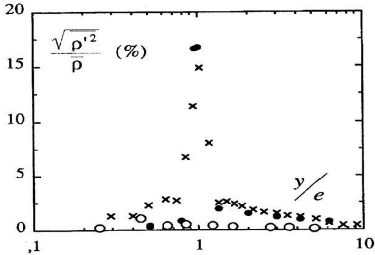
Fig. 2: Profils de fluctuations de densité mesurées par la sonde d'interférence à 1 mm en aval de l'injection d'hélium. x: T_{\text{fil}} = 250\text{ °C} , T_{\text{film}} = 100\text{ °C} , •: T_{\text{fil}} = 75\text{ °C} , T_{\text{film}} = 175\text{ °C} o: LaRue et Libby [2]
