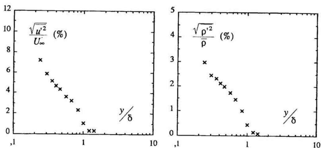
Fig. 4: Profil de fluctuations de vitesse et de densité mesurées par la sonde d'interférence à 10 mm en amont de l'injection d'hélium. U_\infty = 11,6 \text{ m/s} , X_{air\infty} = 0,8 ; T_{fil} = 250^\circ\text{C} , T_{film} = 100^\circ\text{C}
