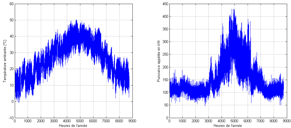
Fig. 3 Représentation de la puissance appelée et de la température ambiante.
