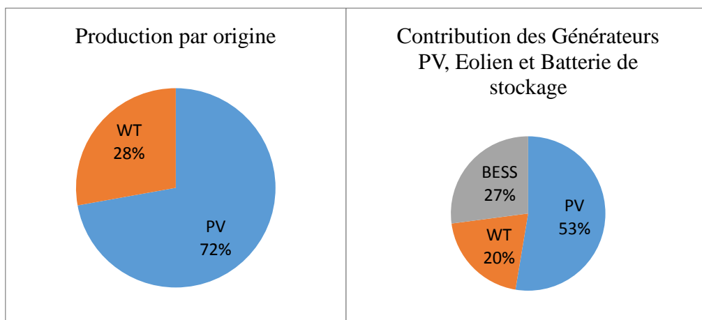
Fig.6 Production annuelle de chaque source
