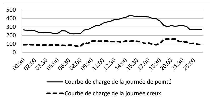
Fig.1 Courbe de charge de M'Guiden (2013).
