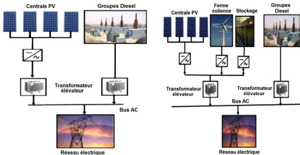
Fig. 2 Architecture d'hybridation diesel-PV et diesel-PV-Eolien avec stockage (Idda et al., 2015).
