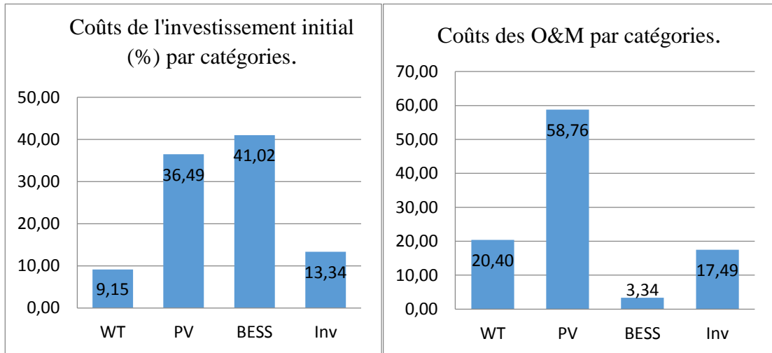
Fig.5 Coûts de l'investissement initial et coûts des O&M par catégories
