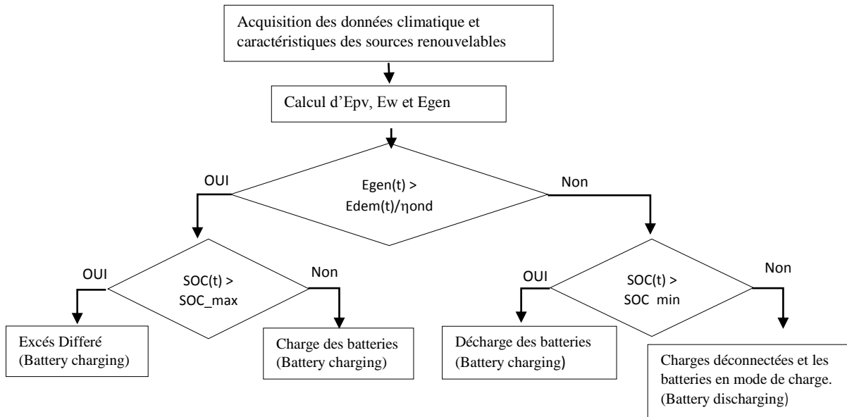
Fig. 2 Stratégie de gestion de l'énergie
