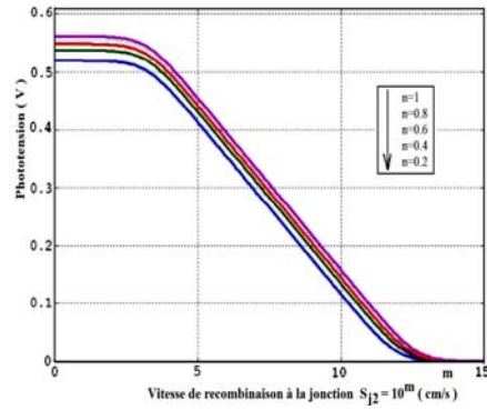
Fig. 13: Photo tension en fonction de la vitesse de recombinaison S_{f2} pour différentes valeurs de n , D=26 \text{ cm}^2/\text{s} , S_{b1}=1000 \text{ cm/s} , H=0.03 \text{ cm} Eclairage par la face avant
