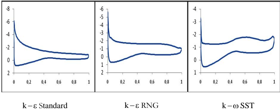
Fig. 5: Coefficients de pression en fonction de la position x/c pour \alpha = 15^\circ
