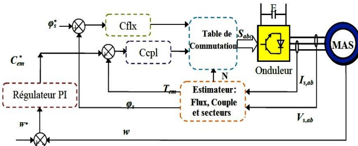
Fig. 1: Schéma structurel du contrôle direct du couple
