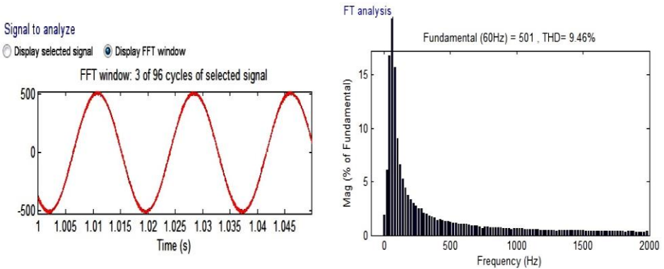
a- THD de courant statorique ( I_{as} )
