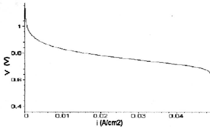
Fig. 4: Courbe caractéristique du modèle électrochimique
