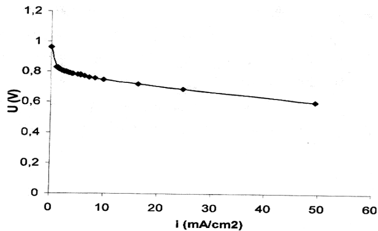
Fig. 5: Courbe caractéristique U = f(i)
