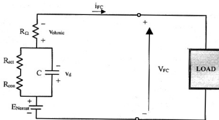
Fig. 2: Schéma électrique dynamique équivalent d'une pile (M.G. Simoes, 2004)
