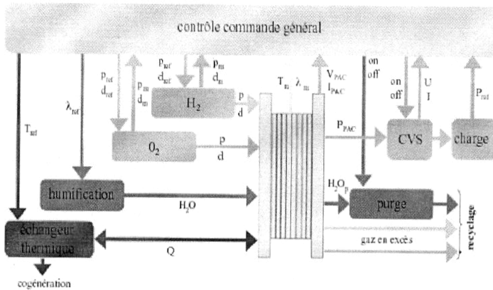
Fig. 3: Schéma général de mise en œuvre d'une PaC (R. Saisset, INPT, 2004)
